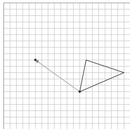
⑥ 平行移動した三角形
